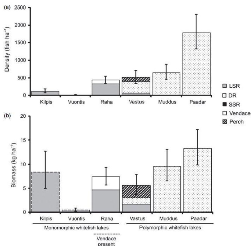
Kuva 4. Siikamuotojen ja muikun keskitiheys ja arvioitu biomassa ulappa-alueella kaikuluotauksen ja troolauksen perusteella. Biomassa-arvioihin Kilpisjärvellä ja Vuontisjärvellä on suhtauduttava pienellä varauksella. Kilpisjärvellä ei ole troolattu, vaan käytetty verkkoja. Selite: LSR on pohjasiika, DR on reeska ja SSR on räpys; Vendace on muikku ja Perch on ahven. (lähde: Malinen ym. 2014).
