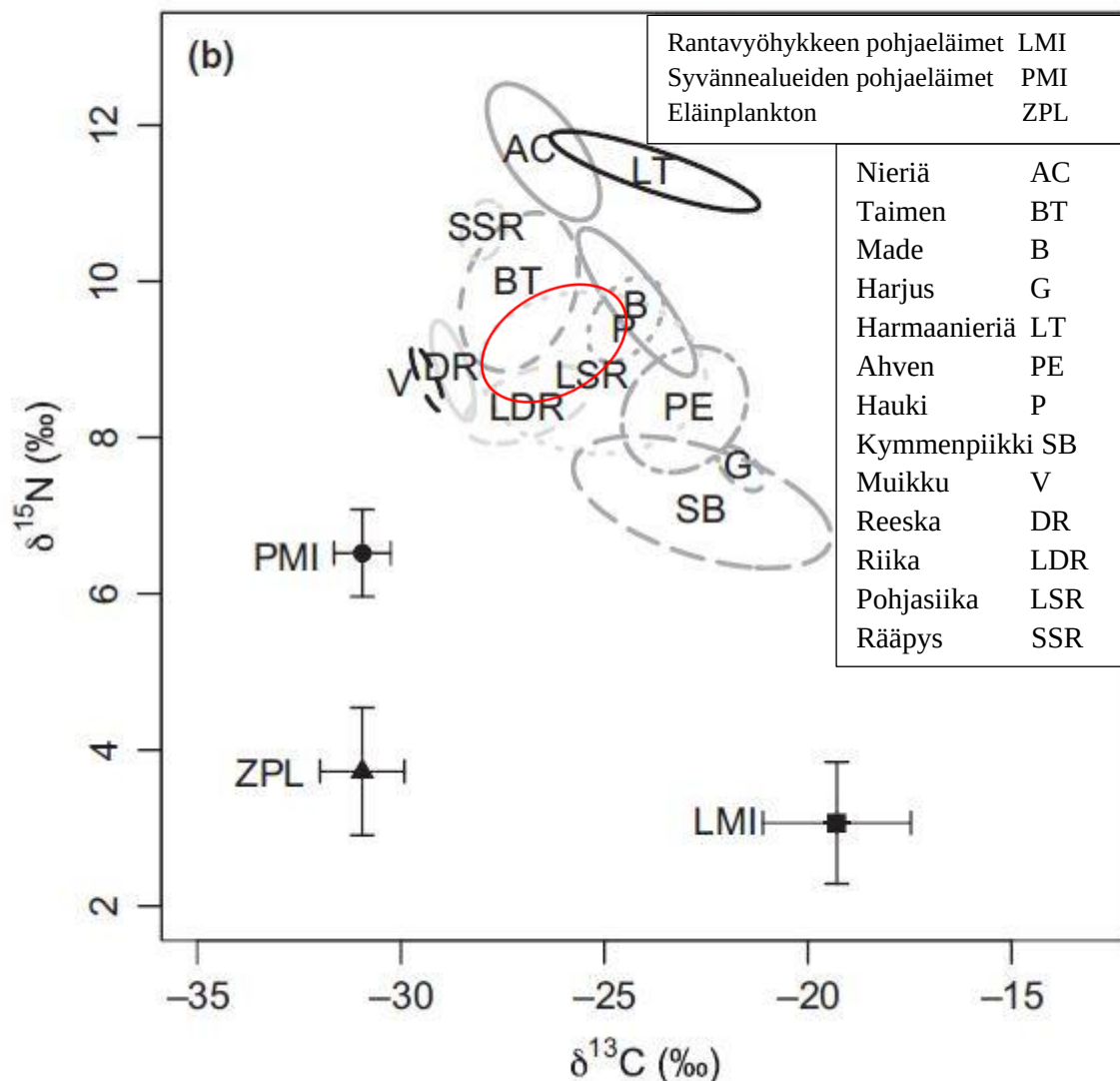
Kuva 3. Inarijärven ravintoverkon rakenne esitettynä hiilen ja typen vakaila isotoopeilla. Hiili kuvastaa paikkaa (vasemmalla on ulappa-alue ja oikealla rantavyöhyke) x-akselilla ja y-akselilla tyyppi kuvaa kalan trofiatasoa ravintoverkossa (saaliskala, petokala). Kalojen ekologisen lokeron koko on
